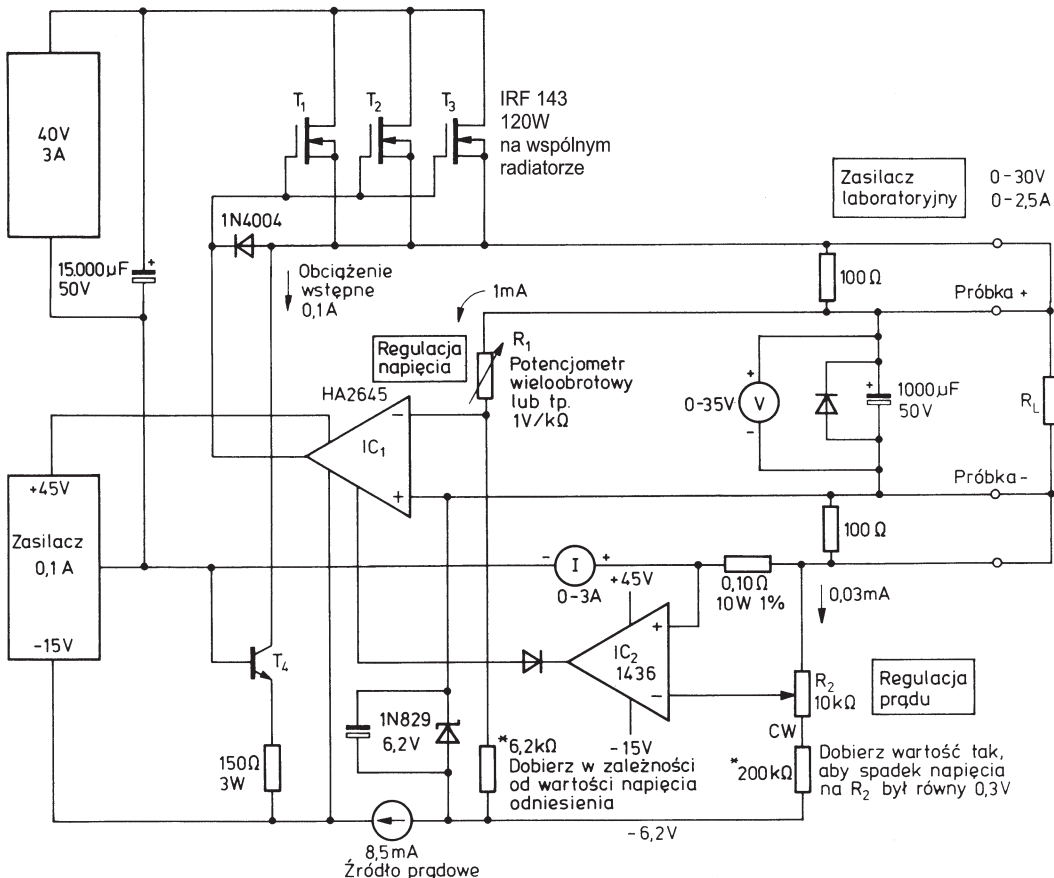
Rysunek 6.16. Laboratoryjny zasilacz stacjonarny
